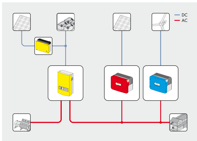
Einphasiges System
